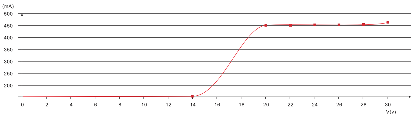
Prąd a długość światła
